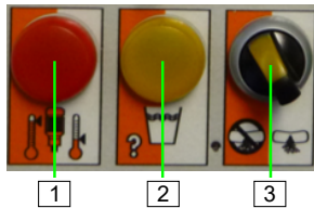
Abb. 77: Störungsanzeigen
