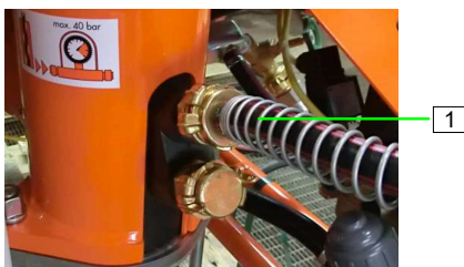
Abb. 71: Wasserschlauch anschließen
