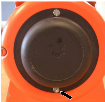
Abb. 85: Öffnung Filterabdeckung
