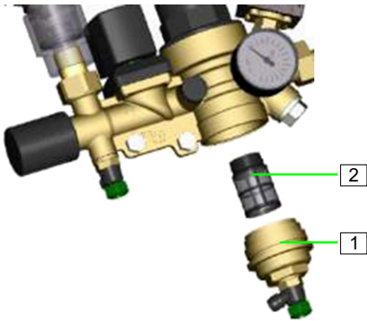
Abb. 87: Schmutzfängersieb
