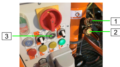
Abb. 38: Mischzone wässern
