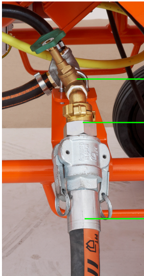
Abb. 39: Mörtelschlauch vorbereiten
