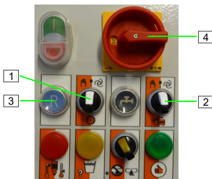
Abb. 78: Rückwärtslauf
