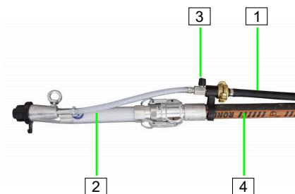
Abb. 43: Spritzgerät
