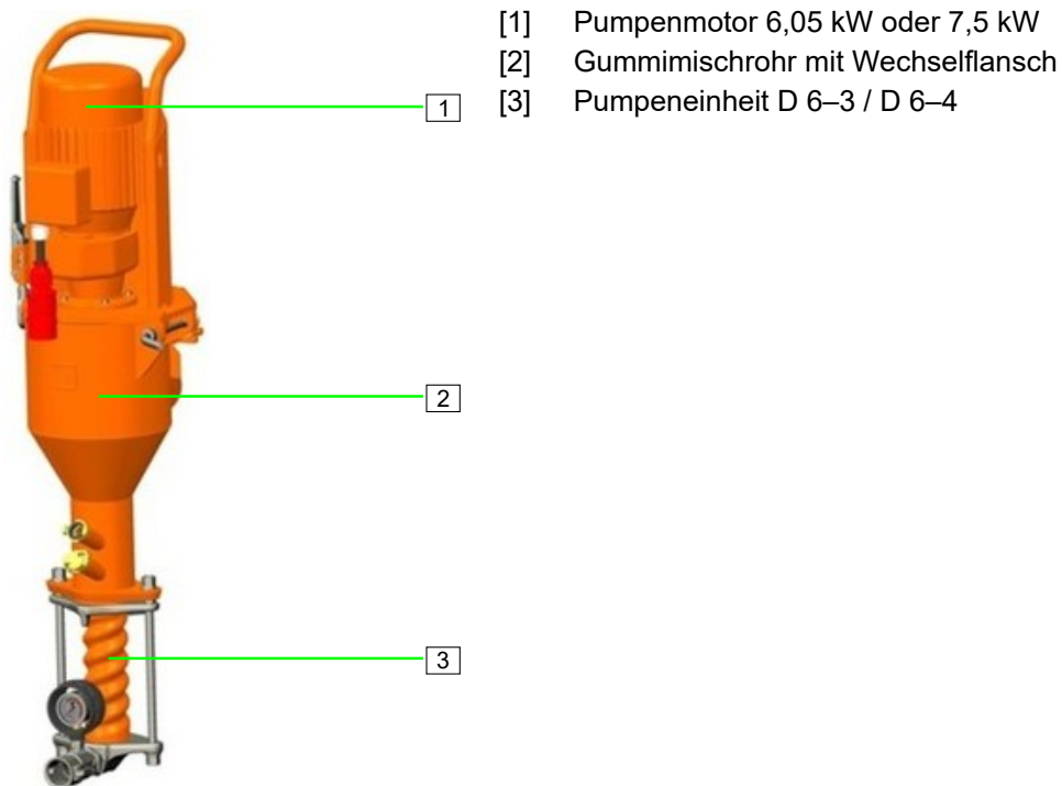
Abb. 13: Baugruppe Mischrohr mit Motor
