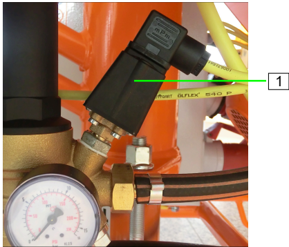
Abb. 88: Druckschalter Wasser
