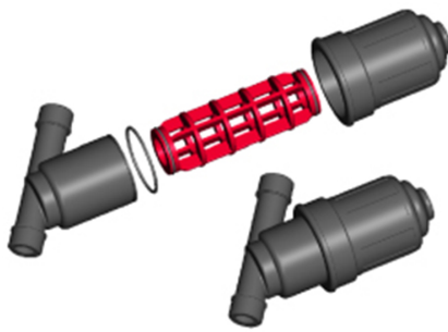
Abb. 63: Schmutzfänger
