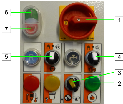
Abb. 81: Maschine wieder einschalten
