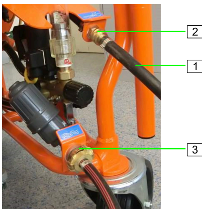
Abb. 64: Luftschlauch anschließen
