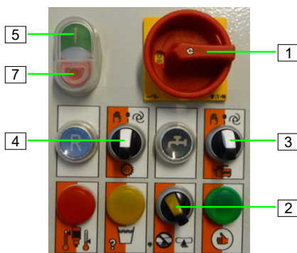
Abb. 49: Maschine einschalten
