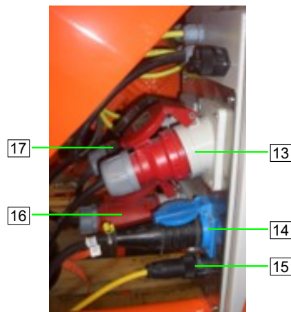
Abb. 12: Baugruppe Schaltschrank
