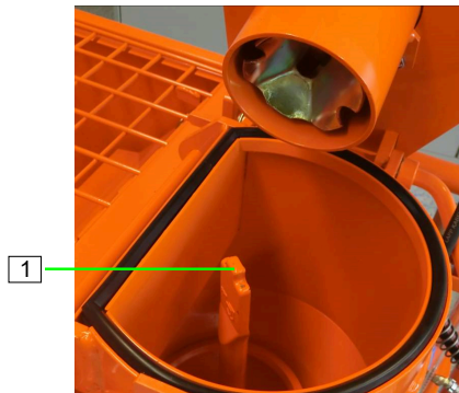
Abb. 72: Motorkippflansch öffnen
