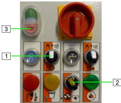
Abb. 67: Mischrohr leer fahren
