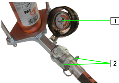
Abb. 68: Mörtelschlauch abkuppeln
