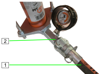
Abb. 40: Mörtelschlauch anschließen
