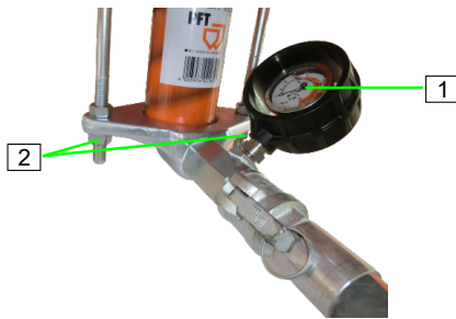
Abb. 79: Mörtdruck überprüfen und ablassen
