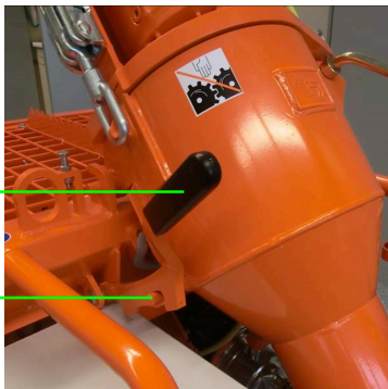
Abb. 91: Mischrohr hochklappen
