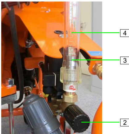
Abb. 37: Wassermenge einstellen
