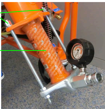
Abb. 92: Pumpe wechseln
