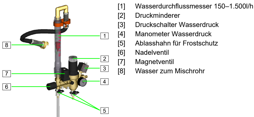
Abb. 14: Baugruppe Wasserarmatur
