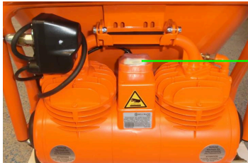
Abb. 44: Luftkompressor einschalten
