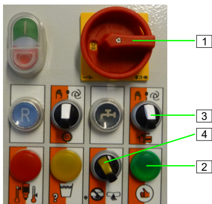
Abb. 35: Maschine einschalten
