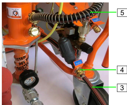
Abb. 32: Wasser anschließen
