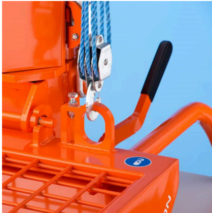
Abb. 5: Anschlagpunkte
