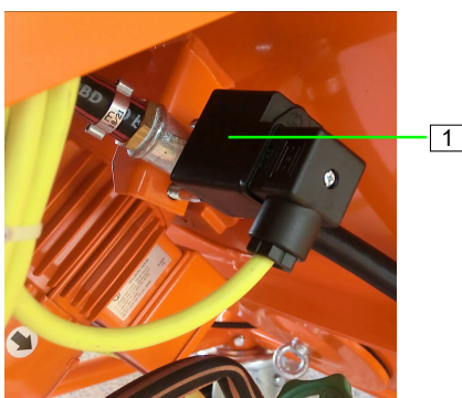
Abb. 89: Druckschalter Luft
